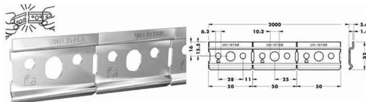
Bevestigingslat type 874
