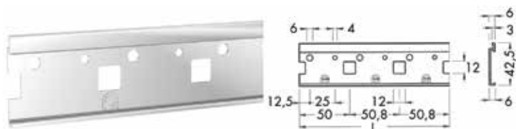
Bevestigingslat type 870/880
