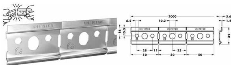
Bevestigingslat type 874
