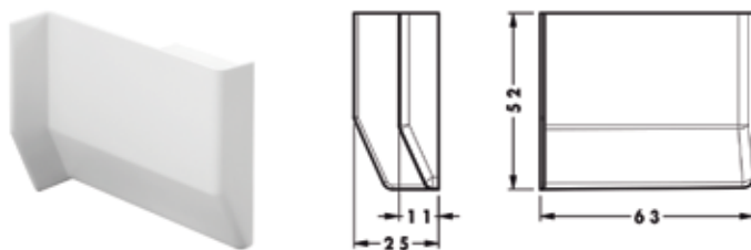
Sierkap voor kastophanger type 701.15.Z1
