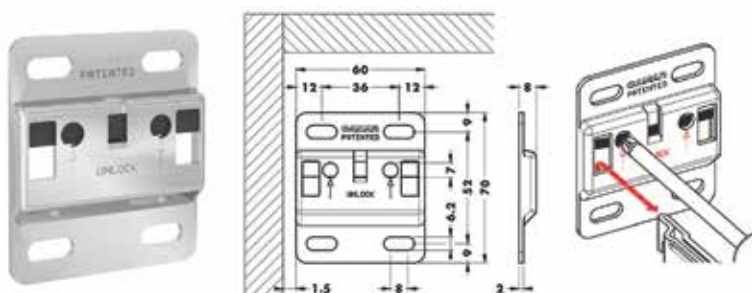
Bevestigingsplaat type 897.AS.Z1.60.70
