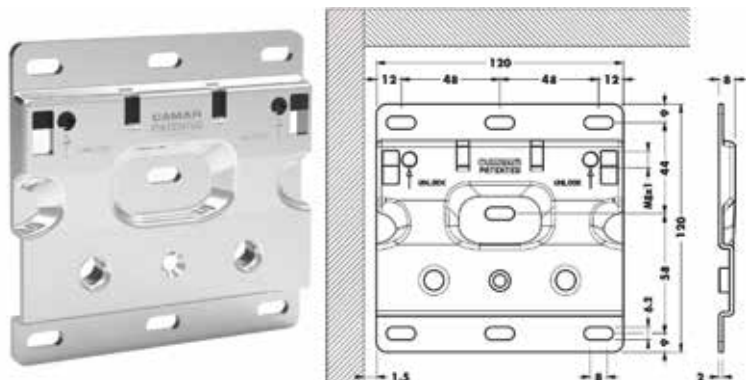
Bevestigingsplaat type 897.AS.Z1.12.12
