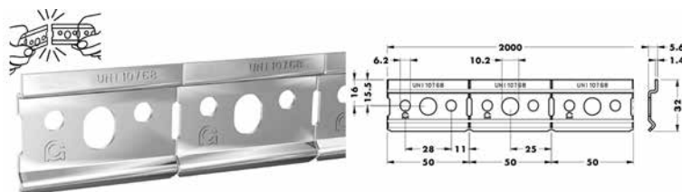
Bevestigingslat type 874.AC.Z1.12.00.05P
