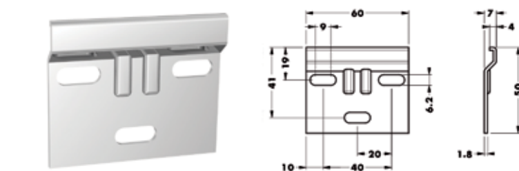
Bevestigingsplaat type 890.AC.00.60.LS
