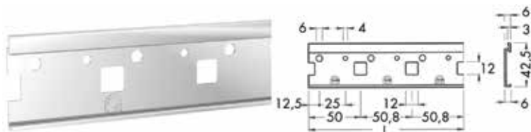
Bevestigingslat type 870/880
