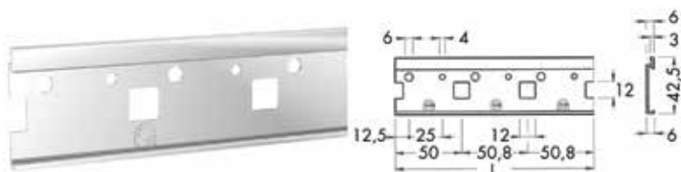
Bevestigingslat type 870/880
